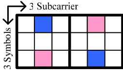
Fig. 9 2-antenna 3x3 tile for 802.16m
