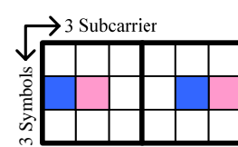
Fig. 5 2-antenna 3x3 tile for 802.16e
