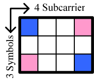
Fig. 4 2-antenna 4x3 tile for 802.16e
