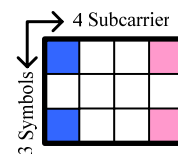
Fig. c 2-antenna 4x3 tile for 802.16m
