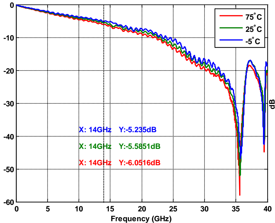
PCBA 1
