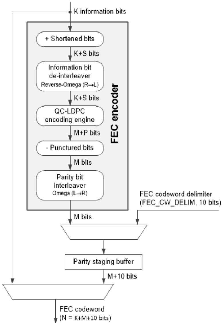
Figure 142-6 LDPC FEC encoder
