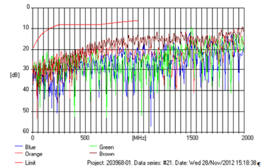
RETURNLOSS-Channel#1-Fromterminalend.f
